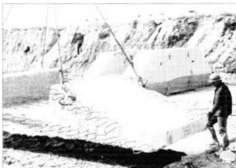
Укладка первых блоков будущей электростанции.
