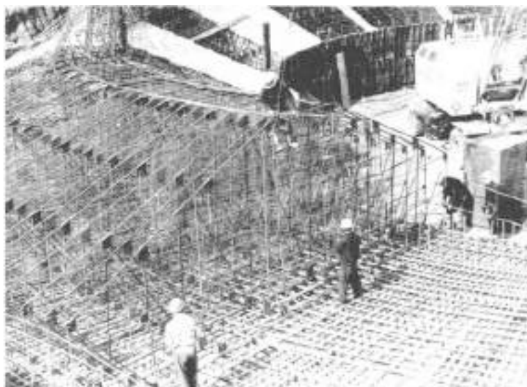
Закладка основания дымовой трубы ГРЭС-1
