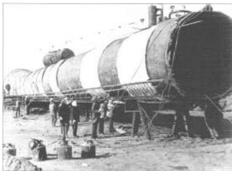
Монтаж пусковой котельной ГРЭС-1
